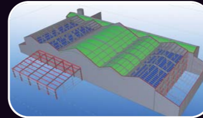
Renforcement bâtiment existant (11)
