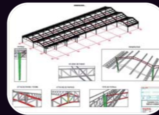
Renforcement bâtiment existant (04)
